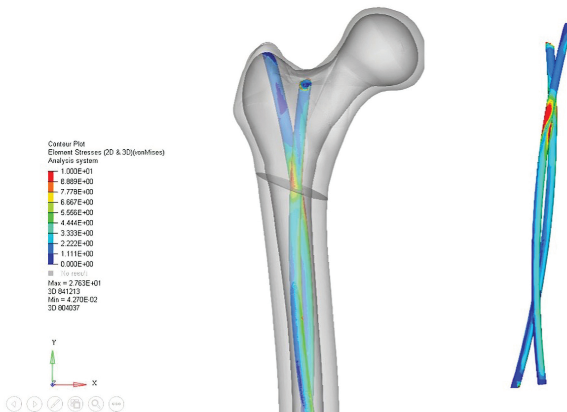
Fig. 2 A figura representa a reconstrução da região proximal do fêmur, o corte da osteotomia e as hastes flexíveis. No detalhe ao lado estão apresentadas as hastes sem o contorno ósseo, ilustrando a concentração das tensões equivalentes de Von Mises que são maiores na região da osteotomia (áreas em vermelho; região crítica). Se houver falência do implante ele vai ocorrer nesse nível, levando à perda da redução.
