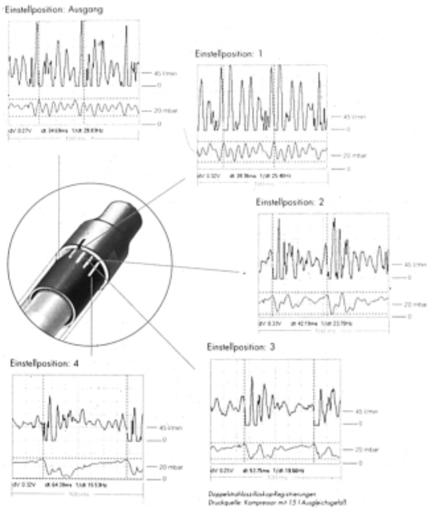
Abb. 2 Druckflussverhalten bei verschiedenen Positionen des RC-Cornet®; Druckquelle: Kompressor mit einem Fluss von 0,75 l/s.
