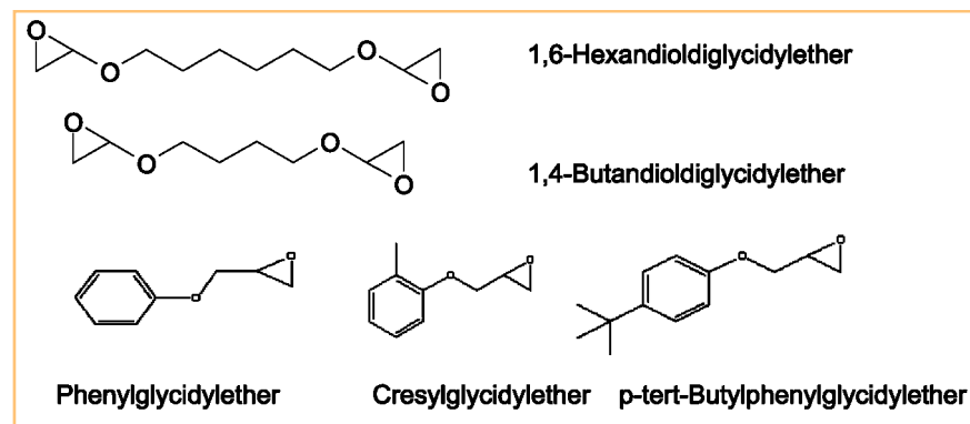
Abb. 1 Chemische Formeln der praxisrelevanten reaktiven Verdünner.
