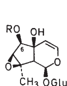
6-seneciolyantirrhinoside (83)
