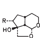
cistanin (45); R = OH cistachlorin (46); R = Cl
