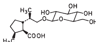
nepetariaside (54)
