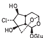
cistanin (45); R = OH cistachlorin (46); R = Cl
